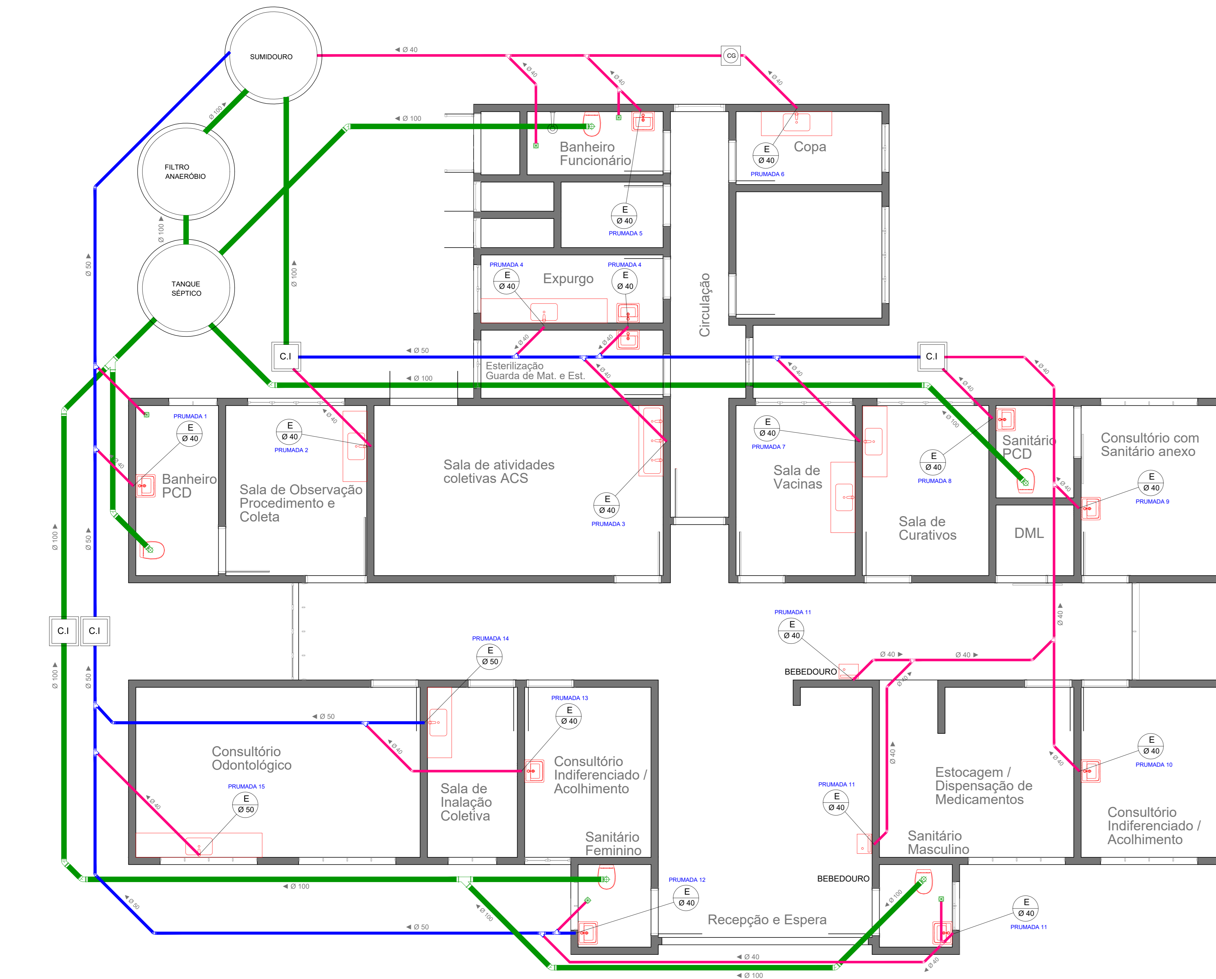
PLANTA BAIXA - REDE DE ESGOTO - ESC 1/40
