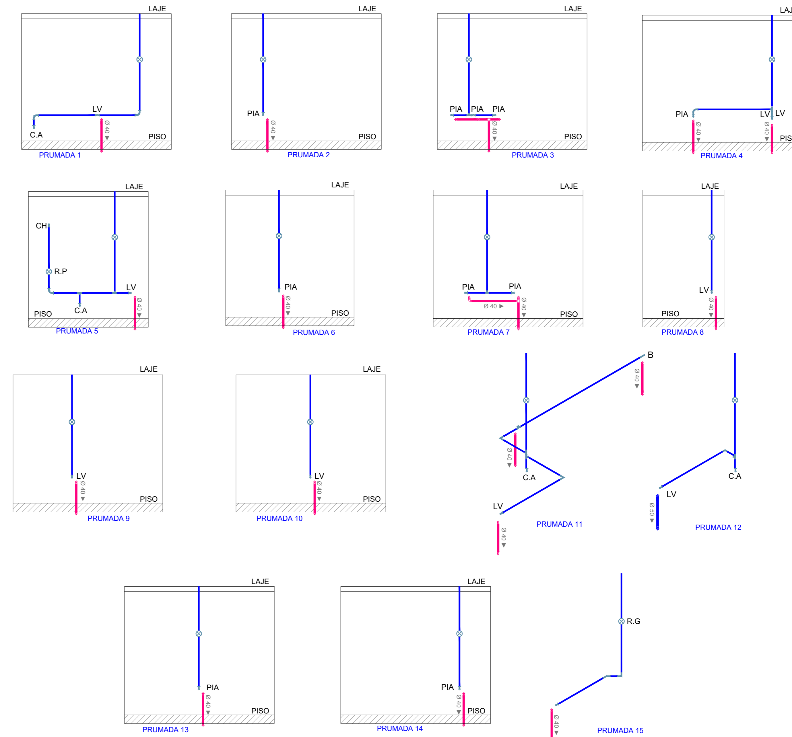
PRUMADAS - ESC. 1/50
