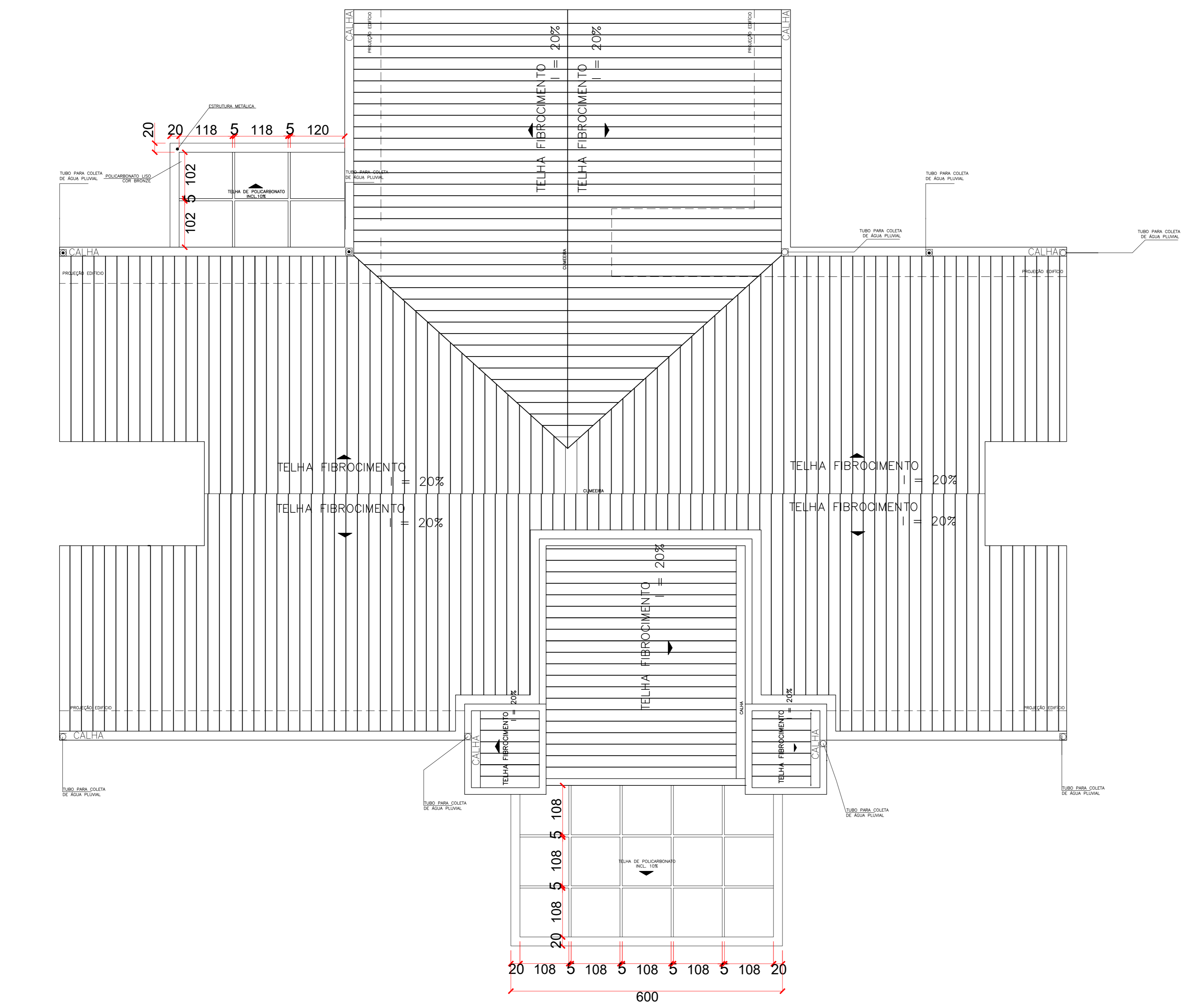
PLANTA DE COBERTURA - ESC 1/50
