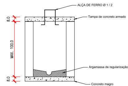
Corte A-A' escala 1:15
