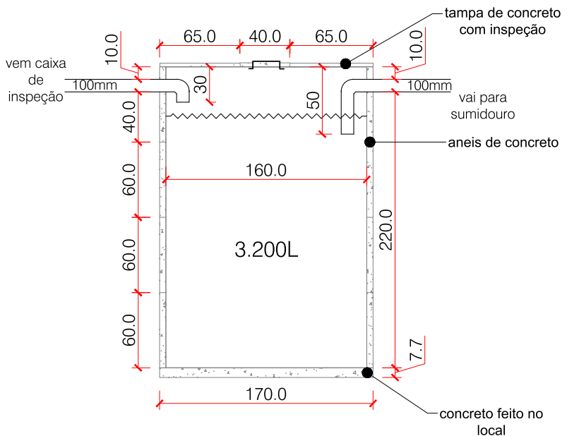
FS - TANQUE SÉPTICO escala 1:15
