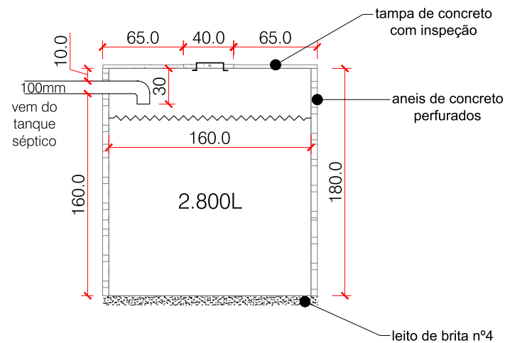
SM - SUMIDOURO escala 1:15
