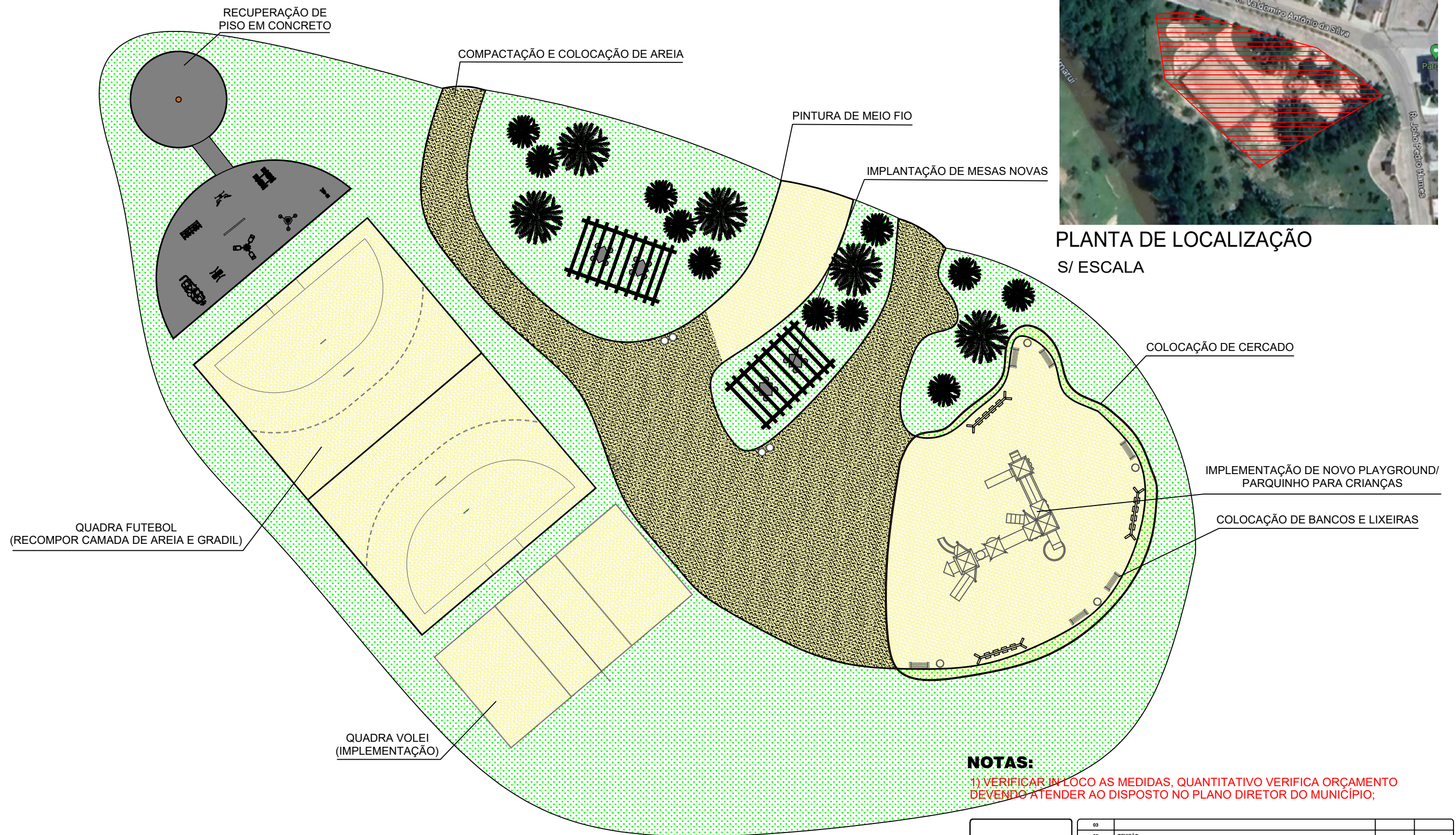
PLANTA BAIXA S/ ESCALA
